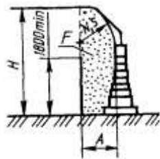
а) жесткое ограждение
