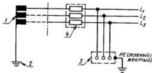
1 - точка заземления энергосистемы; 2 - земля; 3 - открытые проводящие части; 4 - реактор ограничения тока нулевой последовательности; L_1, L_2, L_3 - фазные проводники энергосистемы; PE - защитный проводник
