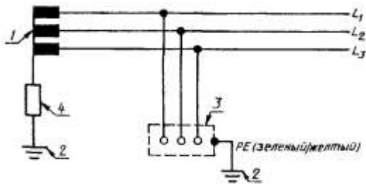
1 - точка заземления энергосистемы; 2 - земля; 3 - открытые проводящие части; 4 - заземляющее сопротивление (резистор или реактор); L_1, L_2, L_3 - фазные проводники энергосистемы; PE - защитный проводник
