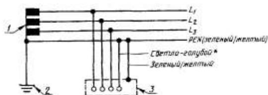
Рисунок 7 - Энергосистема TN с отдельным нулевым проводником и защитными проводниками в энергосистеме
