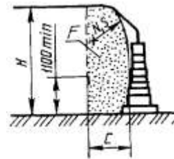
с) ограждение с поручнями, цепями или канатом
